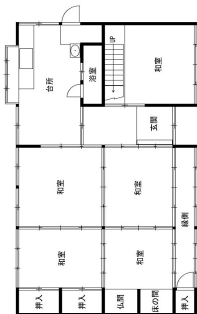
1階平面図
