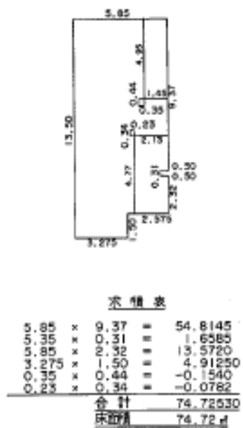
専有部分平面図
