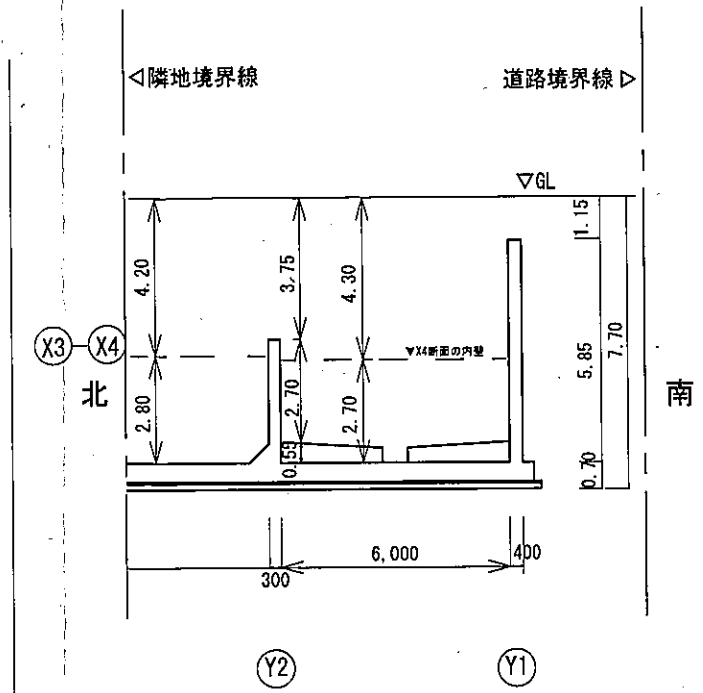
《断面図(X軸断面矢視)》 X3-X4
