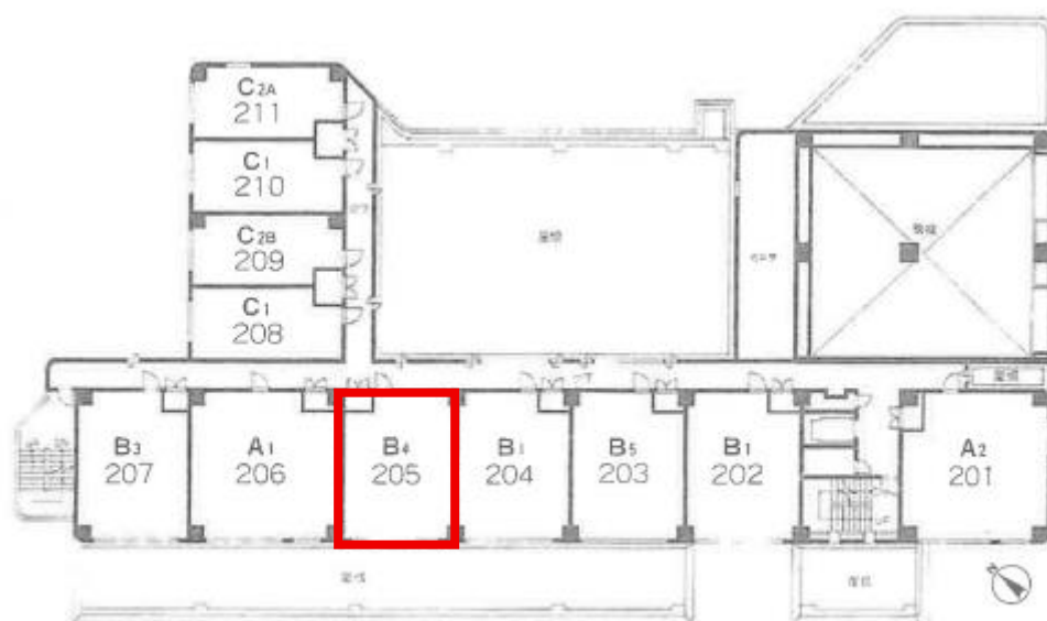
2階平面図
